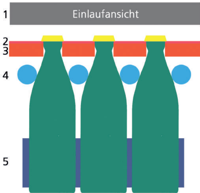
1 Magnetband 2 Abhebemesser 4 Flaschen-Niederhalterung (einstellbar)
